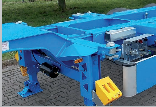
2 Strang - Mittenausschub
